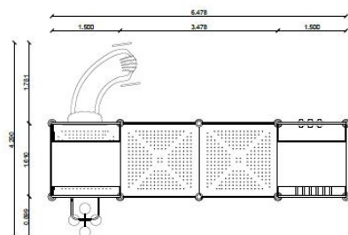
VISTA SUPERIOR Escala 1:80
