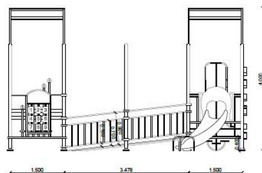
VISTA LATERAL Escala 1:80
