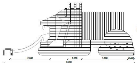
VISTA LATERAL Escala 1:50
