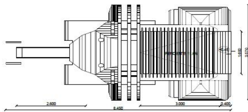
VISTA SUPERIOR Escala 1:50
